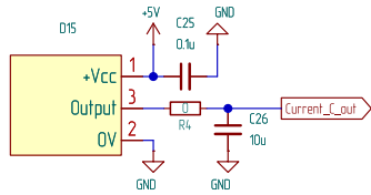
Датчик тока фазы С
