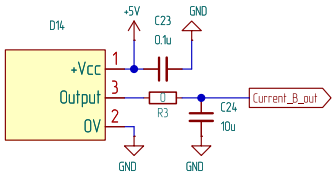
Датчик тока фазы В
