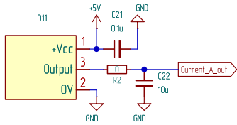
Датчик тока фазы А
