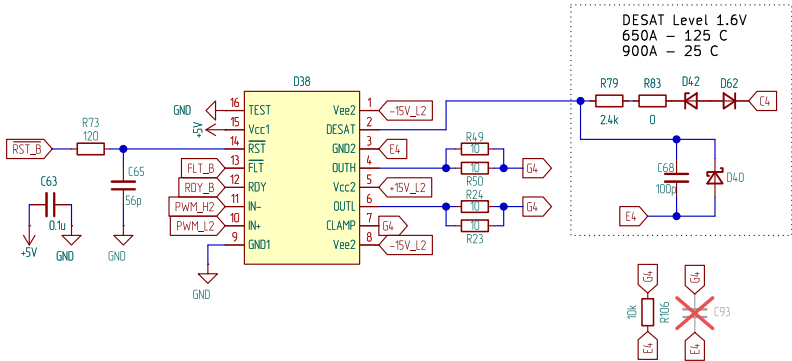
Драйвер нижнего ключа фазы В
