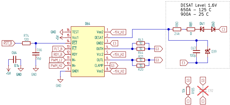
Драйвер верхнего ключа фазы В
